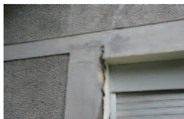
구조체 균열 및 콘크리트 파손, 탈락
